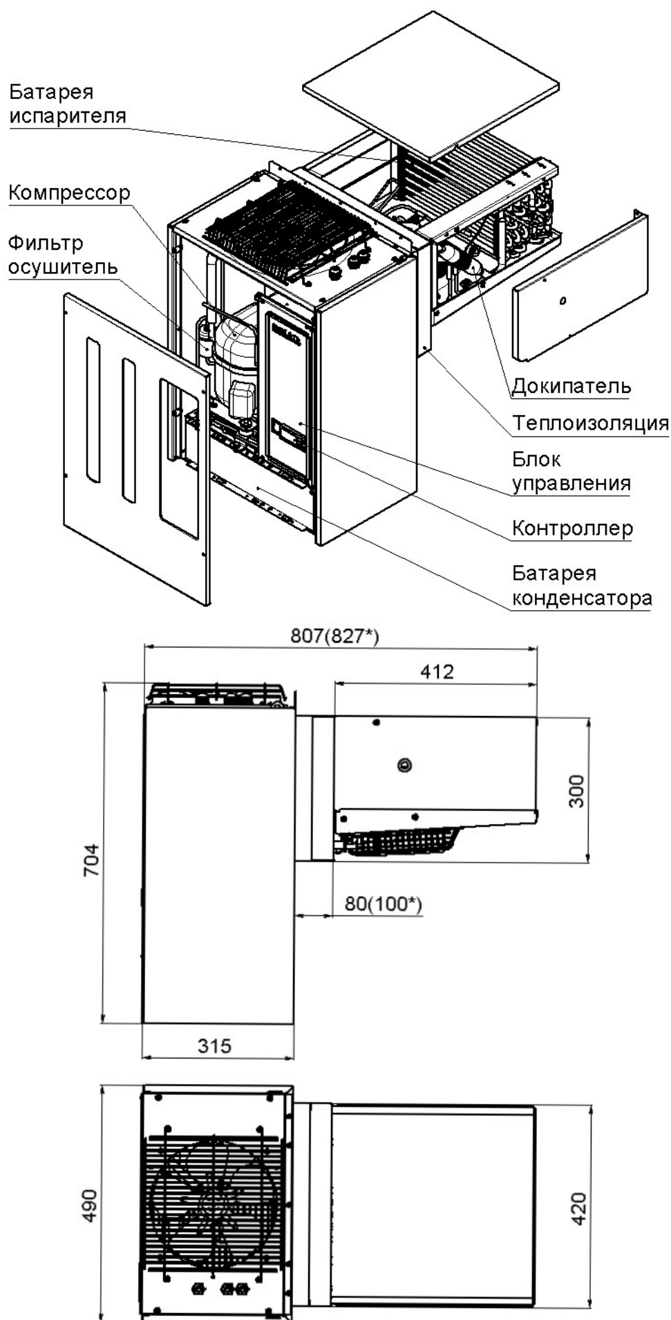
Рис.1 Общий вид и габаритные размеры холодильной машины (моноблока) 121 серии: * - Низкотемпературные холодильные машины
